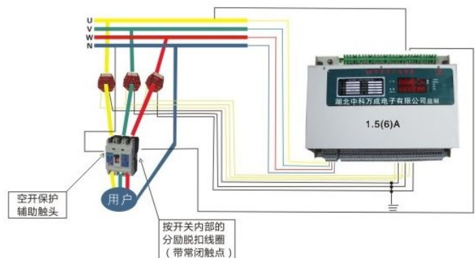
预付费接线示意图(接分励脱扣器)
